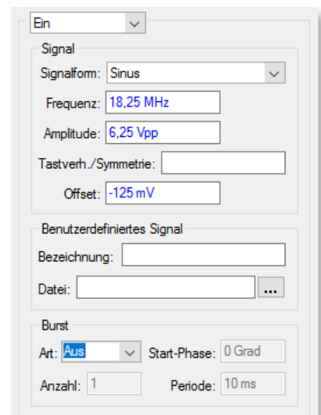
Einstellungen Kurvenformgenerator
