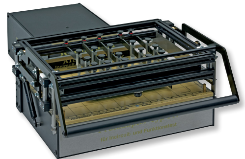
ATS-UKMFT 627 mit Prüfadapter Typ 147
