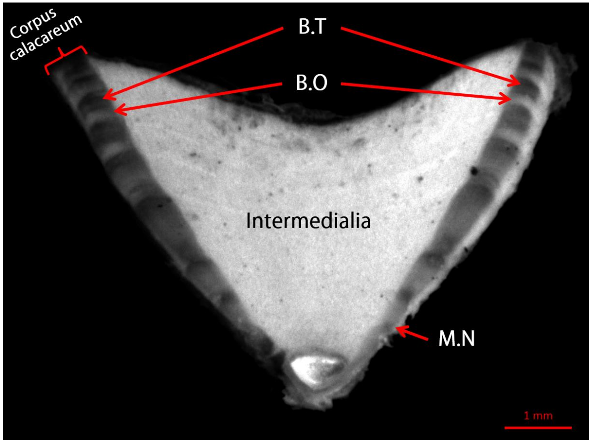
Figura 3. Corte de una vértebra de Mustelus californicus observado con luz reflejada. Bandas opacas (B.O). Bandas traslúcidas (B.T). Marca de nacimiento (M.N).
