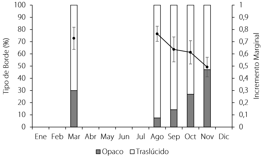
Figura 10. Tipo de borde e incremento marginal de las vértebras de Mustelus californicus para las capturas en el área de Bahía Tortugas B.C.S.
