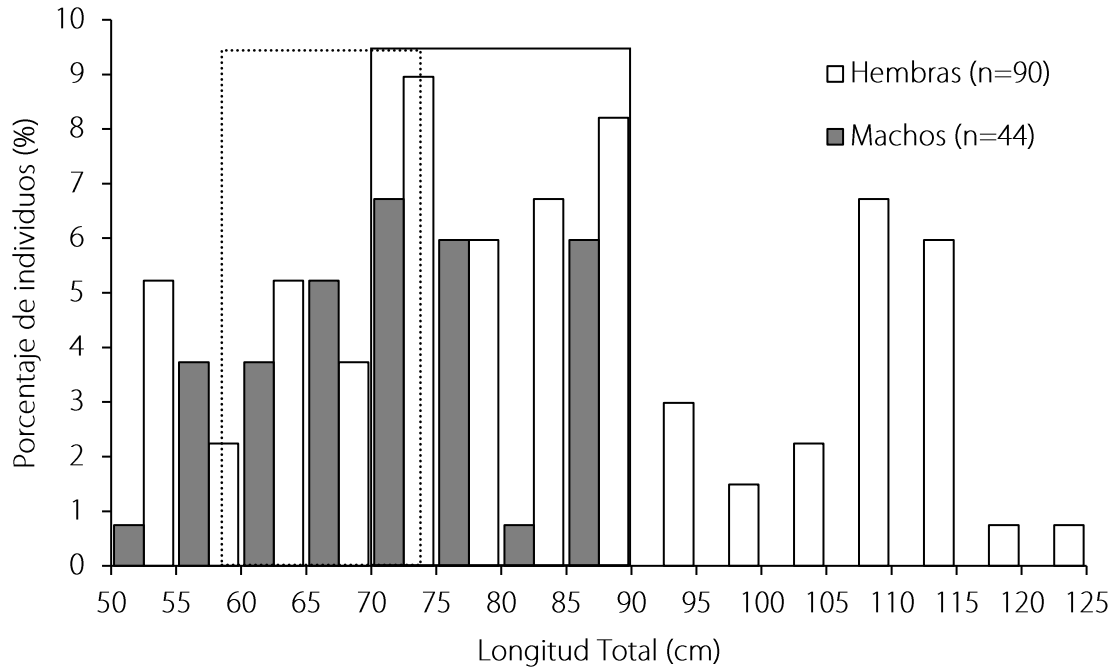
Figura 7. Estructura de tallas por sexos de Mustelus californicus para las capturas en el área de Bahía Tortugas. Intervalos de talla de madurez para machos (línea punteada) y hembras (línea continua) tomados de Compagno (1984) y Pérez-Jiménez (2006).
