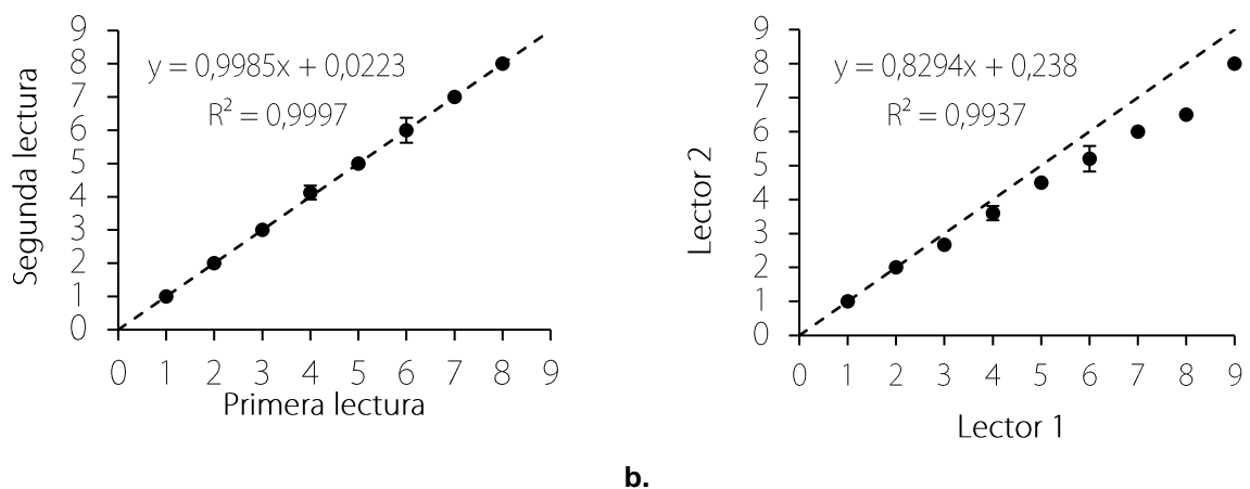
Figura 9. Gráfica de sesgo entre las lecturas hechas por el mismo lector (a) y entre lectores (b).
