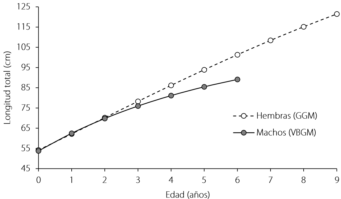
Figura 15. Patrones de crecimiento de machos (VBGM) y hembras (GGM) de Mustelus californicus para el área de Bahía Tortugas, B.C.S.
