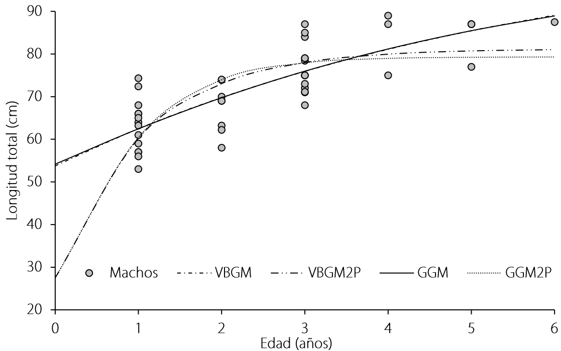
Figura 14. Modelos de crecimiento aplicados a los datos de captura de machos de Mustelus californicus en el área de Bahía Tortugas.
