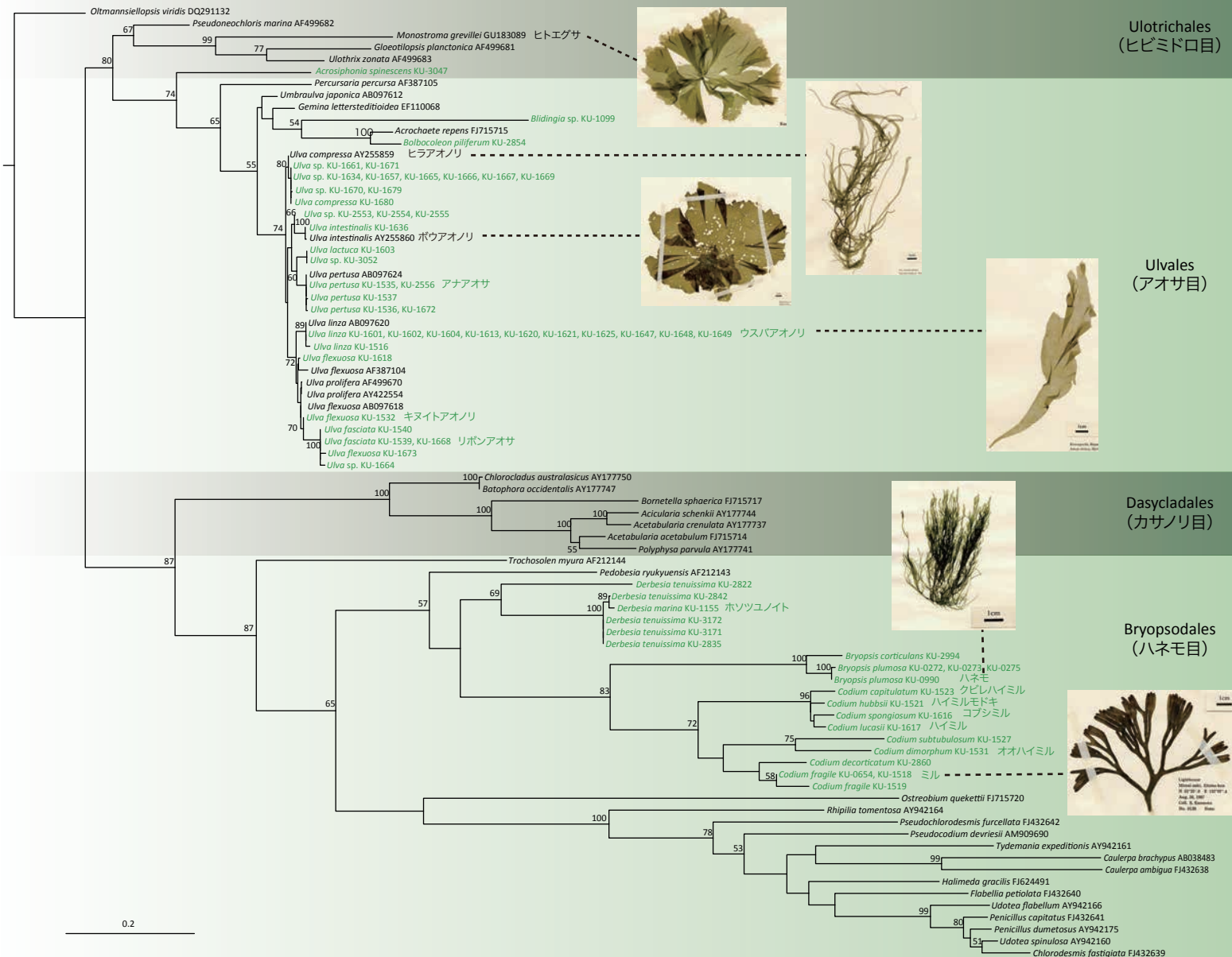
rbcL 遺伝子に基づく分子系統樹 / Molecular phylogenetic tree based on rbcL gene sequence 緑文字 / Green letters : KU-MACC 株 / KU-MACC strains
