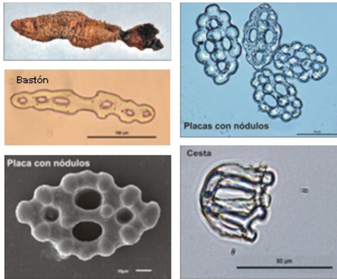
Figura 11. Aslia lefevrii . Morfología externa y cuerpos calcáreos.
