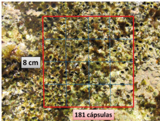
Figura 2. Costra de Dendropoma cristatum . Crust of Dendropoma cristatum .
