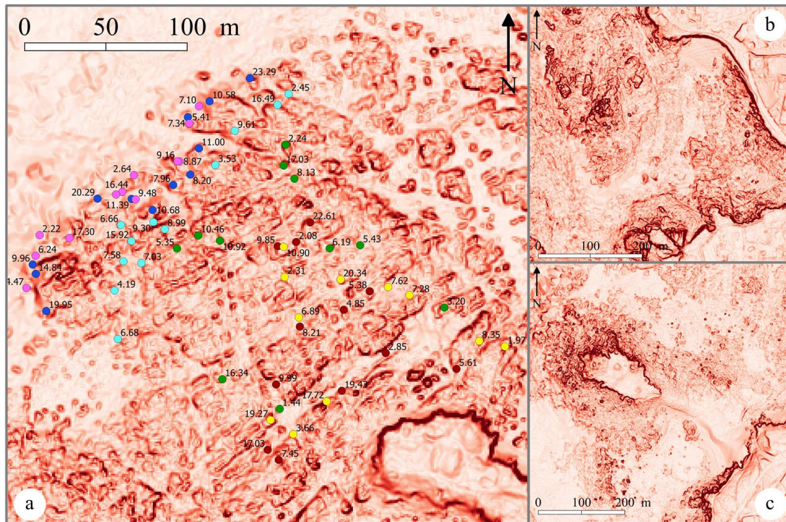
Figure 28 : Pente en degrés déterminée par SIG sur les trois sites échantillonnés pour le chapitre 1. a : Porsal, b :Porspoder, c : île Ségale
