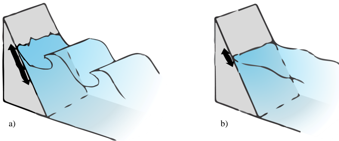
Figure 14 : la zone humidifiée (double flèche noire) est plus étendue dans des zones exposées de par l'action des vagues et les embruns (a) que dans des zones abrités (b). Les zones exposées subissent moins les effets de la dessiccation (adapté de Raffaelli et Hawkins, 1999).
