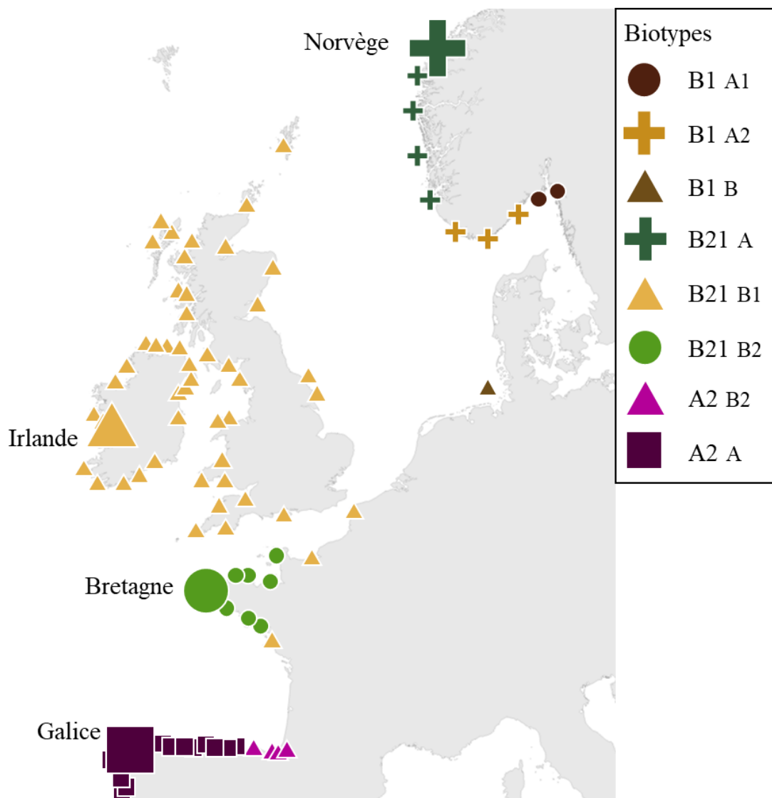
Figure 56 : Classification biologique le long des côtes européennes (biotype), basée sur les données physiques et sur la répartition des espèces de macroalgues d'après Ramos et al. (2014). Les formes colorées agrandies sont situées aux lieux échantillonnés au cours de la thèse (La Galice en 2019, représentée par le biotype A2.A, la Bretagne en 2017, par le biotype B21.B2, l'Irlande en 2018, par le biotype B21.B1, la Norvège en 2019, par le biotype B21.A)
