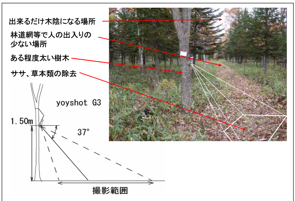
図 4-15 設置仕様
