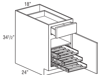
B18CWP18 L or R
