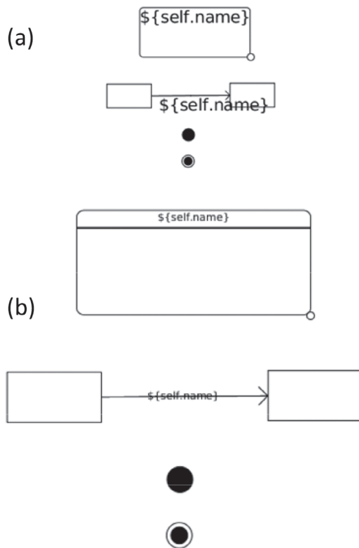
Figura 20. Notación para máquinas de transición de estados.
