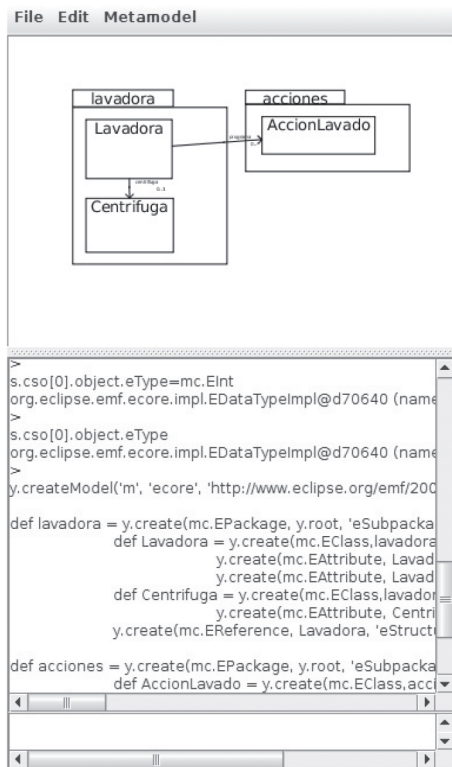
Figura 4. Editor de Modelos. Herramienta de ZoomEnv que permite crear modelos usando la notación definida por el Editor de Sintaxis.
