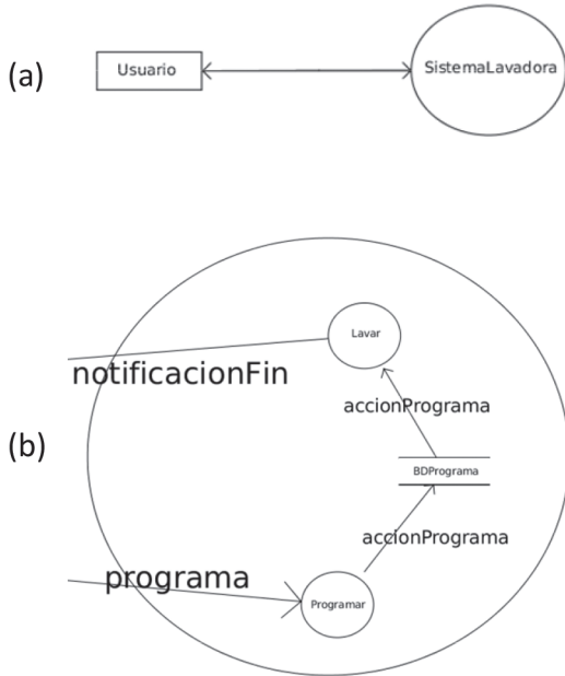
Figura 16. Un diagrama de flujo de datos.
