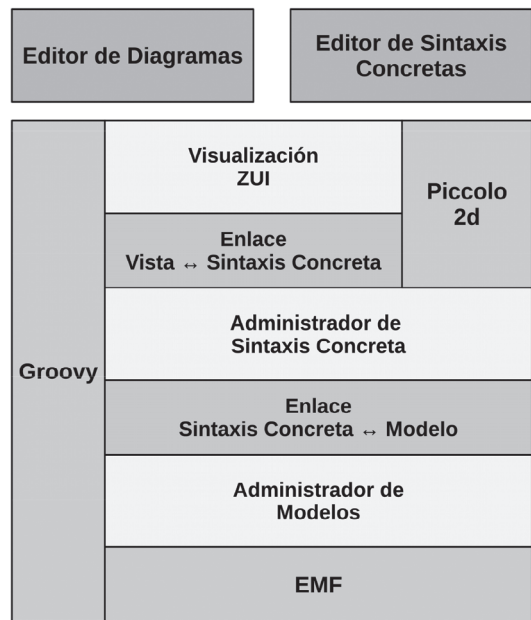
Figura 5. Arquitectura de ZooMEnv. La aplicación comprende una serie de capas de funcionalidad, unificadas a través de un intérprete de lenguaje Groovy.
