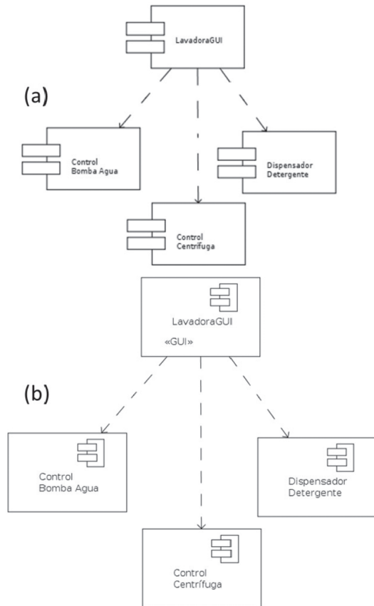
Figura 14. Diagrama de componentes a dos niveles de zoom.
