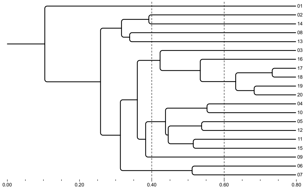
Fig. 4. Similitud florística entre los 20 cuadros en que se dividió la región que comprende el proyecto Flora del Bajío y de regiones adyacentes. Coeficiente de similitud utilizado: Sorensen-Dice; método de agrupamiento: enlace completo.
