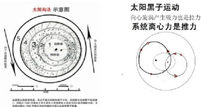
图 2 太阳原始构造物理图像
