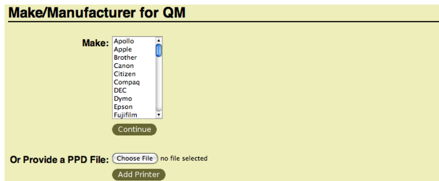
Fig. 40: CUPS - Socket 5
