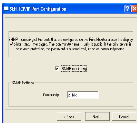
Fig. 14: SEH Print Monitor - SNMP
