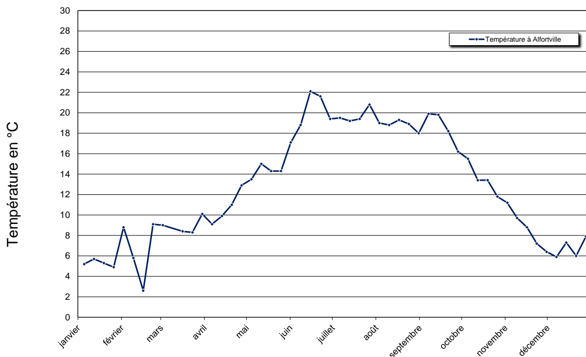
Figure 23 : Température en Marne en 2021
