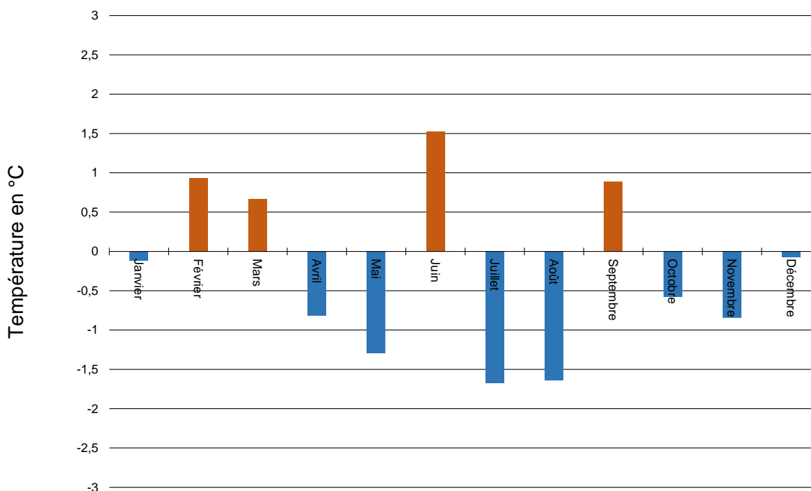
Figure 18 : Différence entre la température moyenne mensuelle en 2021 et la moyenne mensuelle interannuelle de 2006-2020
