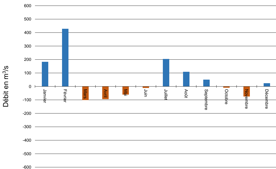
Figure 16 : Différence entre le débit moyen mensuel en 2021 et la moyenne mensuelle interannuelle de 2006-2020
