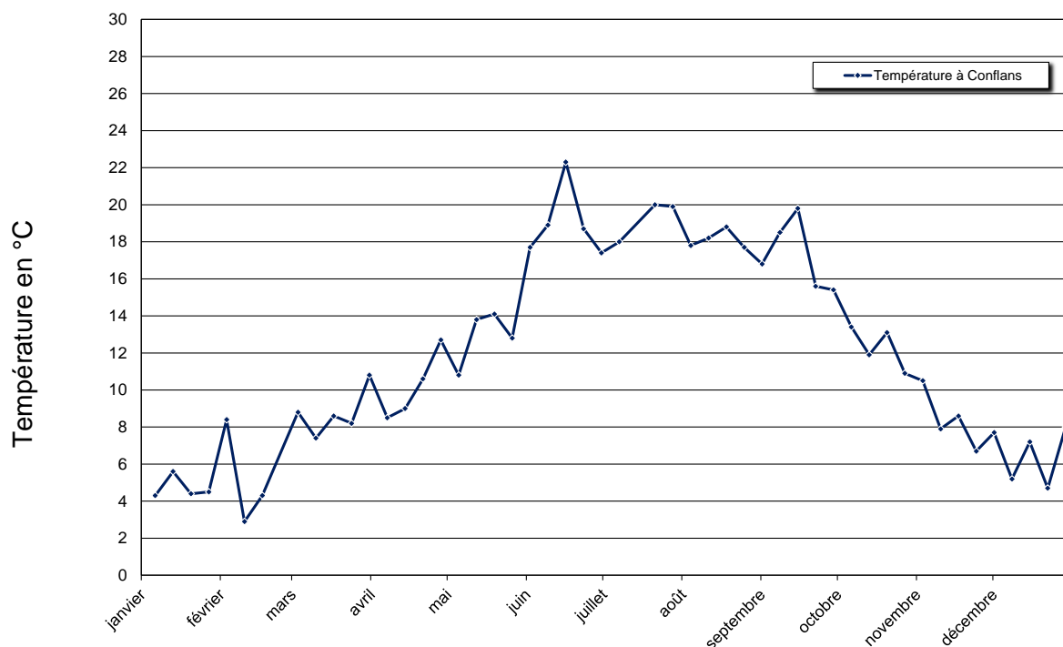
Figure 28 : Température en Oise en 2021
