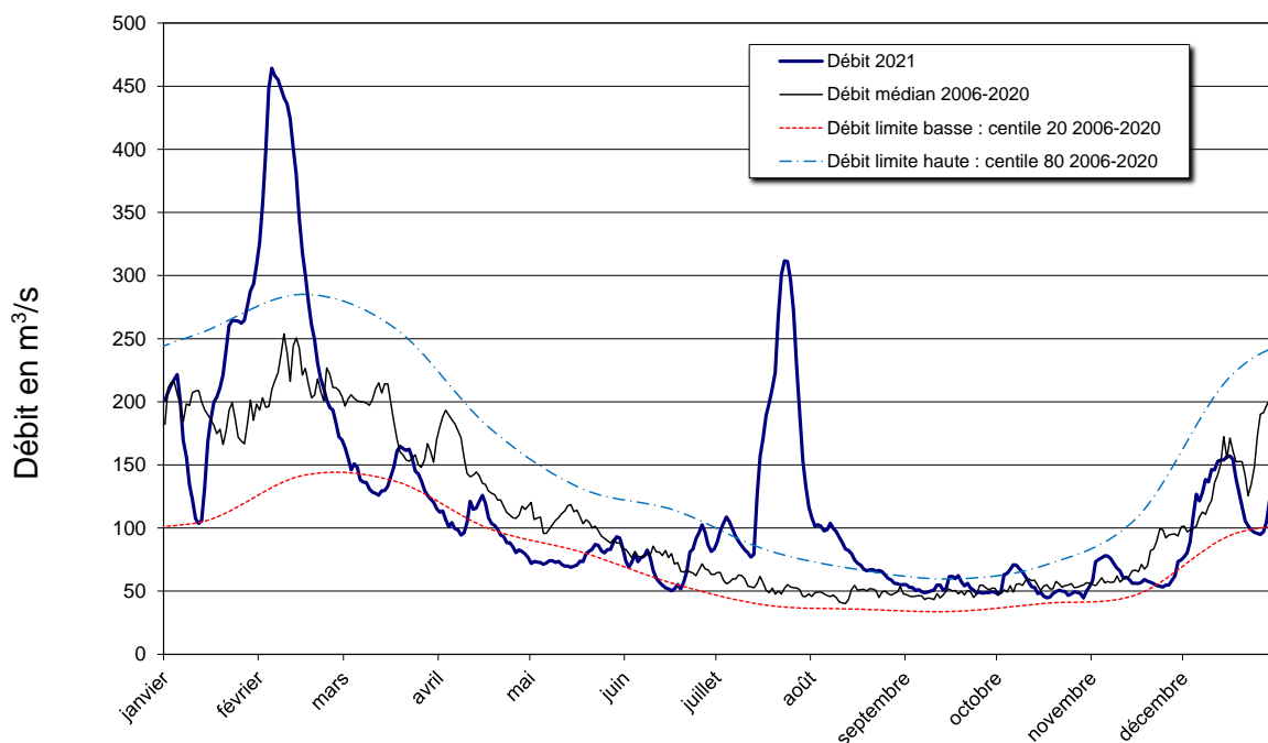
Figure 26 : Débit en Oise en 2021
