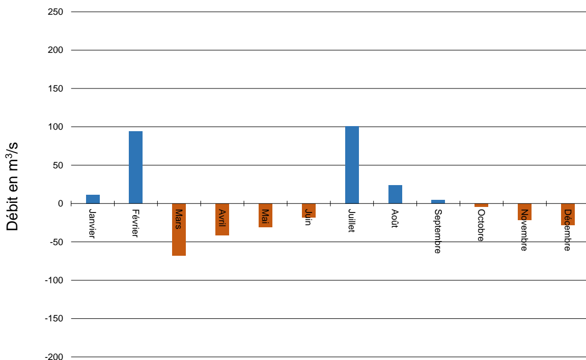
Figure 27 : Différence entre le débit moyen mensuel en 2021 et la moyenne mensuelle interannuelle de 2006-2020
