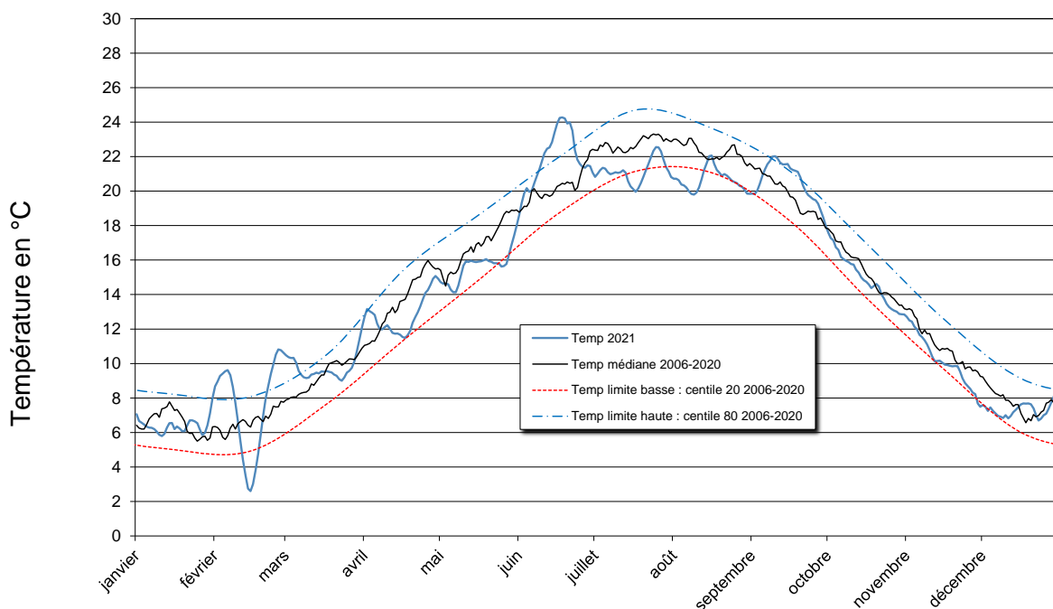
Figure 17 : Température en Seine en 2021
