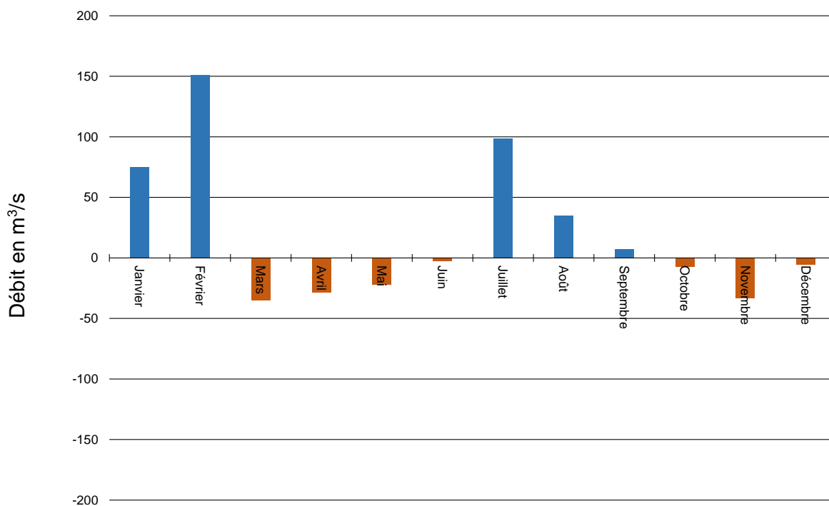
Figure 22 : Différence entre le débit moyen mensuel en 2021 et la moyenne mensuelle interannuelle de 2006-2020
