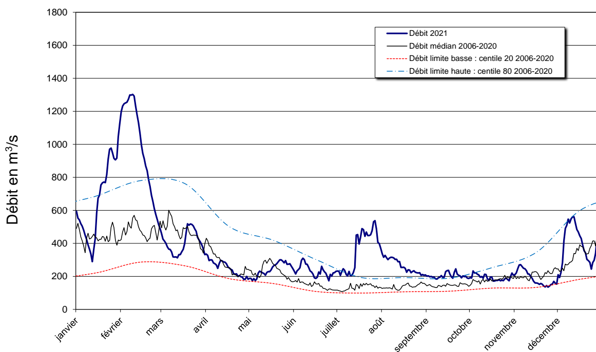
Figure 15 : Débit en Seine en 2021
