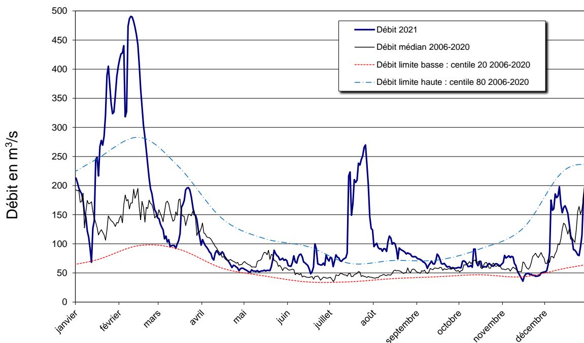
Figure 21 : Débit en Marne en 2021
