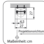
Seitenansicht Gehäuse
