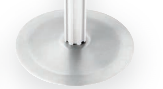
Bezeichnung | Description Größe | Size Art.-Nr. Runder Fuß für Achtkantsäulen, pulverbeschichtetes Stahl ø 300 mm 11 103 Round base for octagonal poles, powder painted steel
