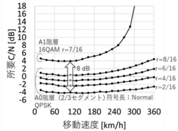
(b) アンテナ 4 本での受信を想定
