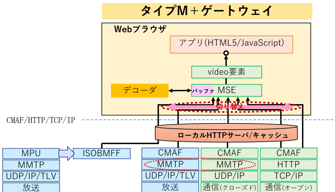
(b) タイプM+ゲートウェイ
