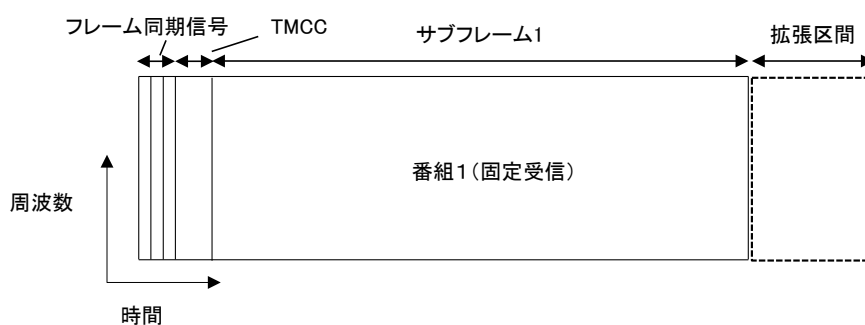
図 4. 1-11 拡張区間を活用する構成例
