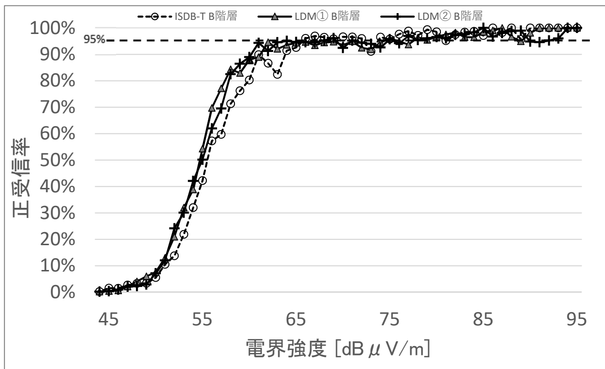
図 7.2-2 正受信率（福岡 LDM 復調器）B 階層
