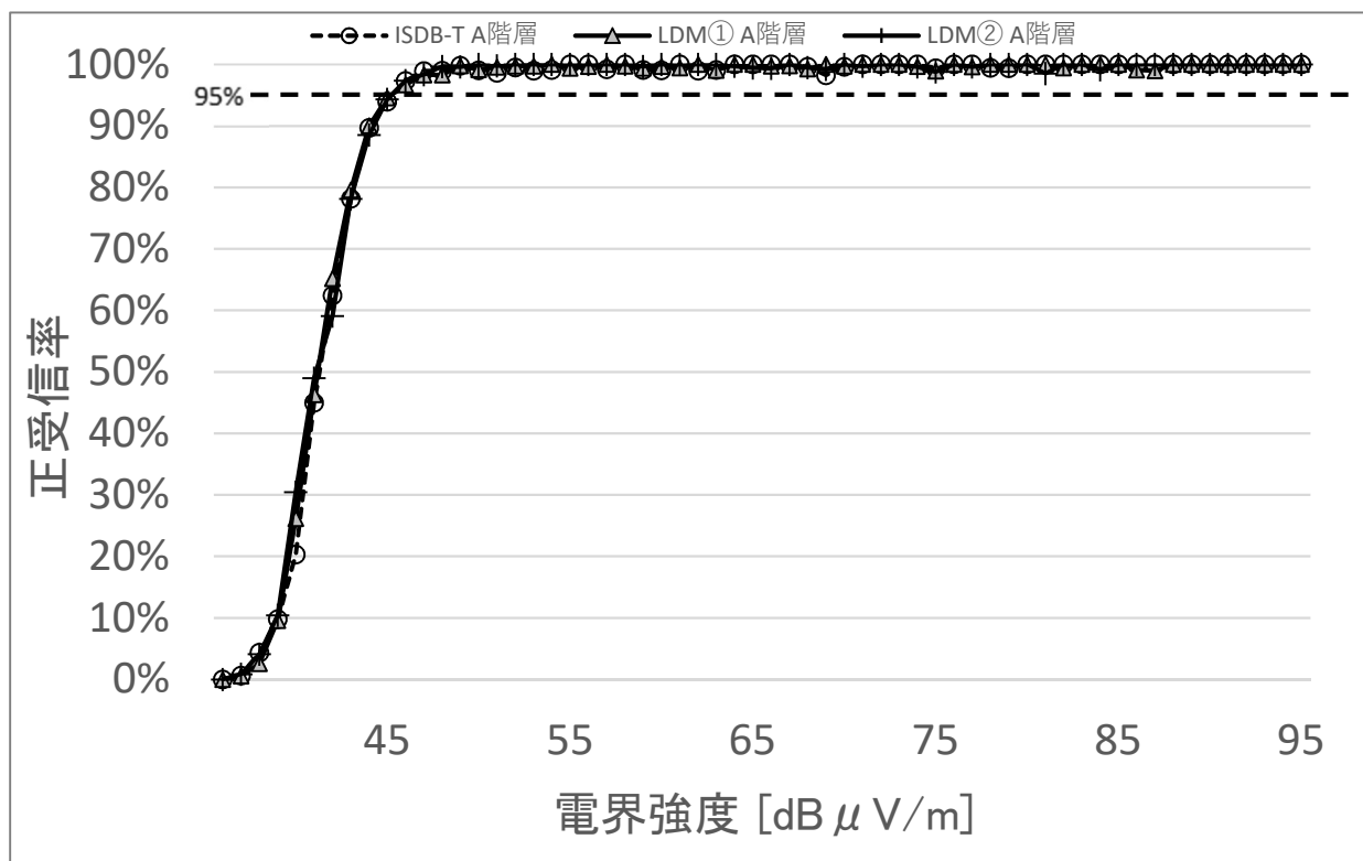
図 7.2-1 正受信率（福岡 LDM 復調器）A 階層
