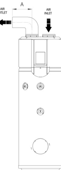
D: Kanalisierte Absonderung ( A \leq 5m )
