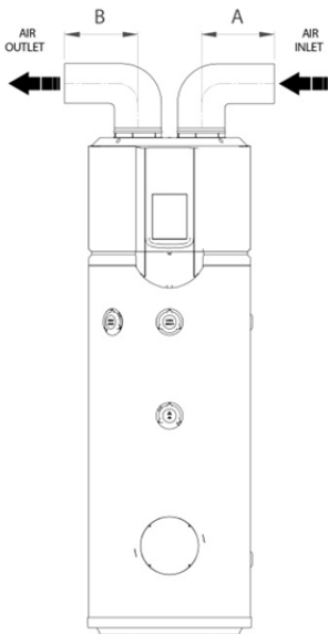
C: Kanalisierte Absaugung und Absonderung ( A+B \leq 5m )
