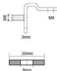
M8 Gewindebolzen Front Terminal
