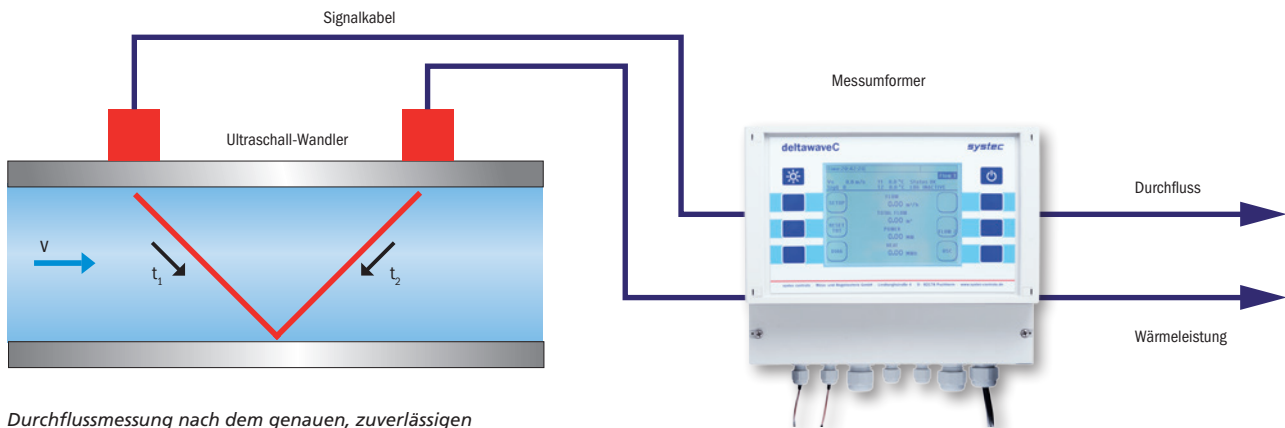
Durchflussmessung nach dem genauen, zuverlässigen Laufzeitdifferenzverfahren – hier im V-Modus
