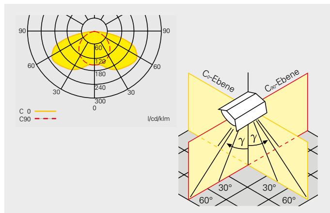
Lichtverteilungskurve (LVK)
