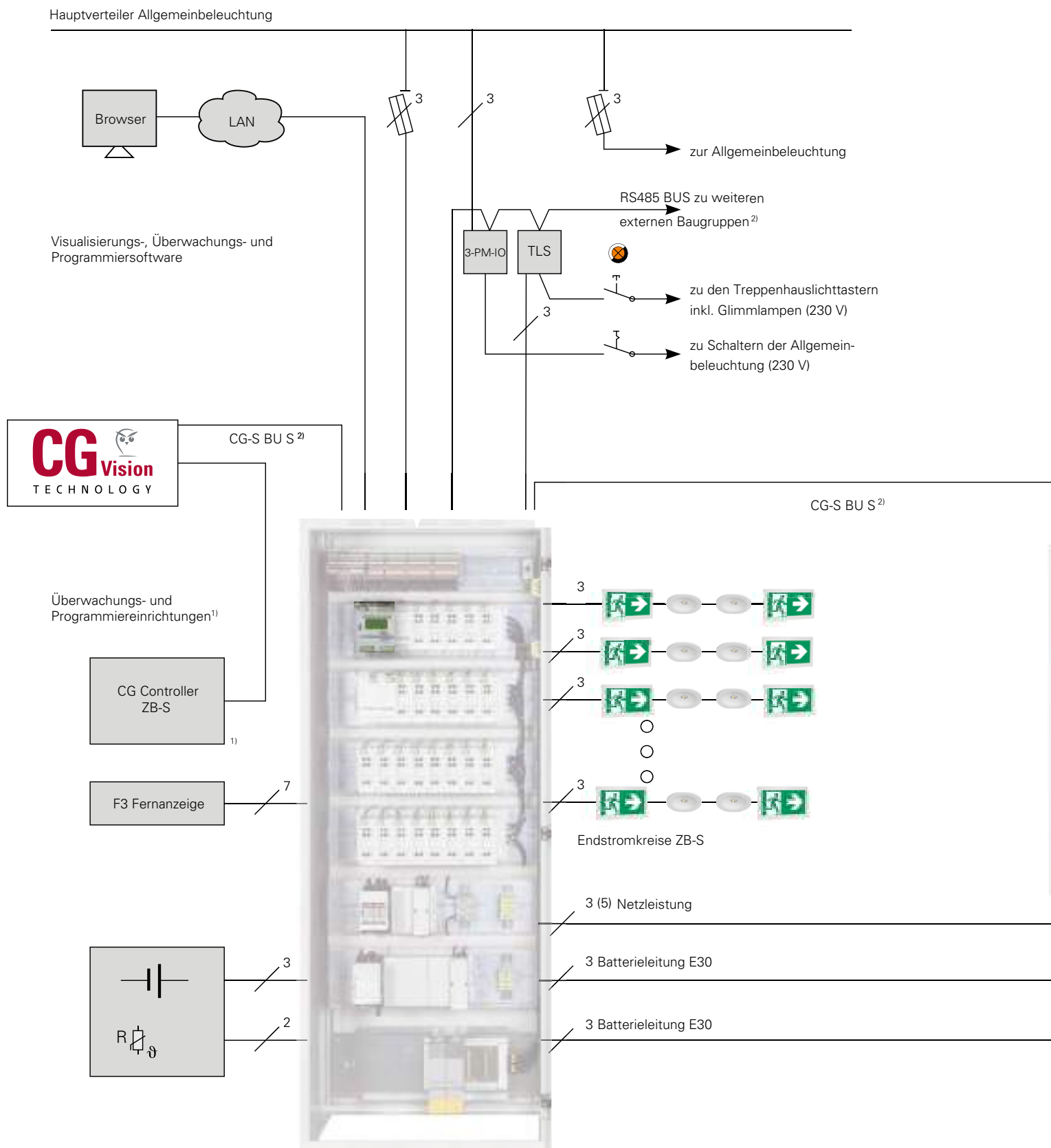
Zentralbatterieanlage ZB-S
