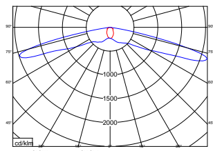
Lichtverteilungskurve HandRail 930x1 LED
