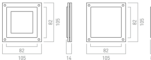
Infomodul Blindmodul
