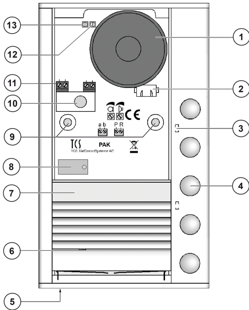
Abb. 1: PAK05-EN ohne Namensschildglas, Frontblende herunter geschoben
