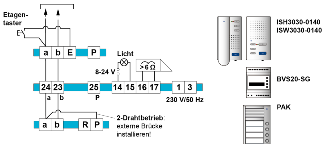
Abb. 5: Schaltungsbeispiel 2-Drahtbetrieb
