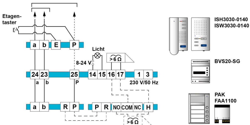
Abb. 4: Schaltungsbeispiel
