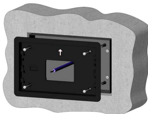
Abb. 5: Montagekasten befestigen
