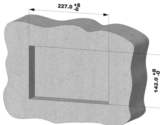
Abb. 2: Maße Wandausschnitt
