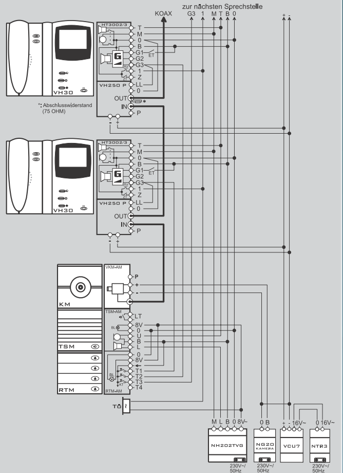
Video-Türsprechanlage mit NH 202 TV G
