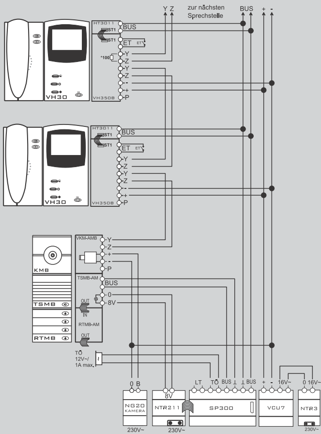
Video-Türsprechanlage BUSTECHNIK/2-Draht-Video
