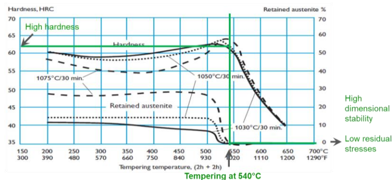
Fig. 4. Dimensional stability Uddeholm Sleipner
