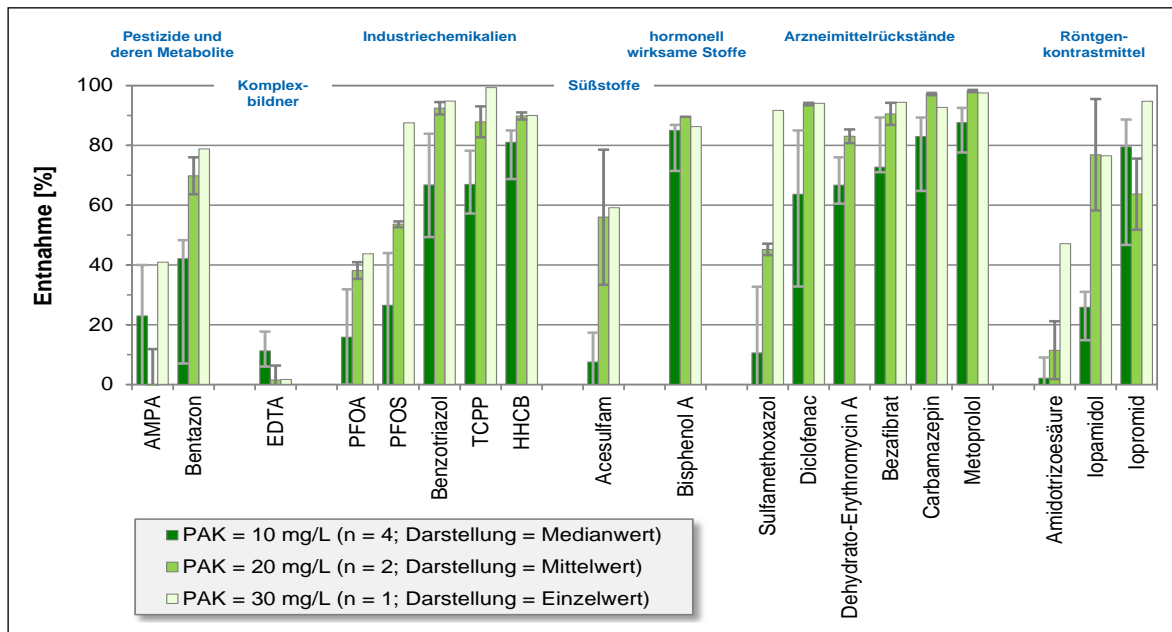
Abbildung 45: Spurestoffentnahme bei unterschiedlichen PAC-Dosiermengen in der Adsorptionsstufe im Klärwerk Mannheim
