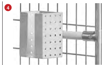
Scannerhalter
