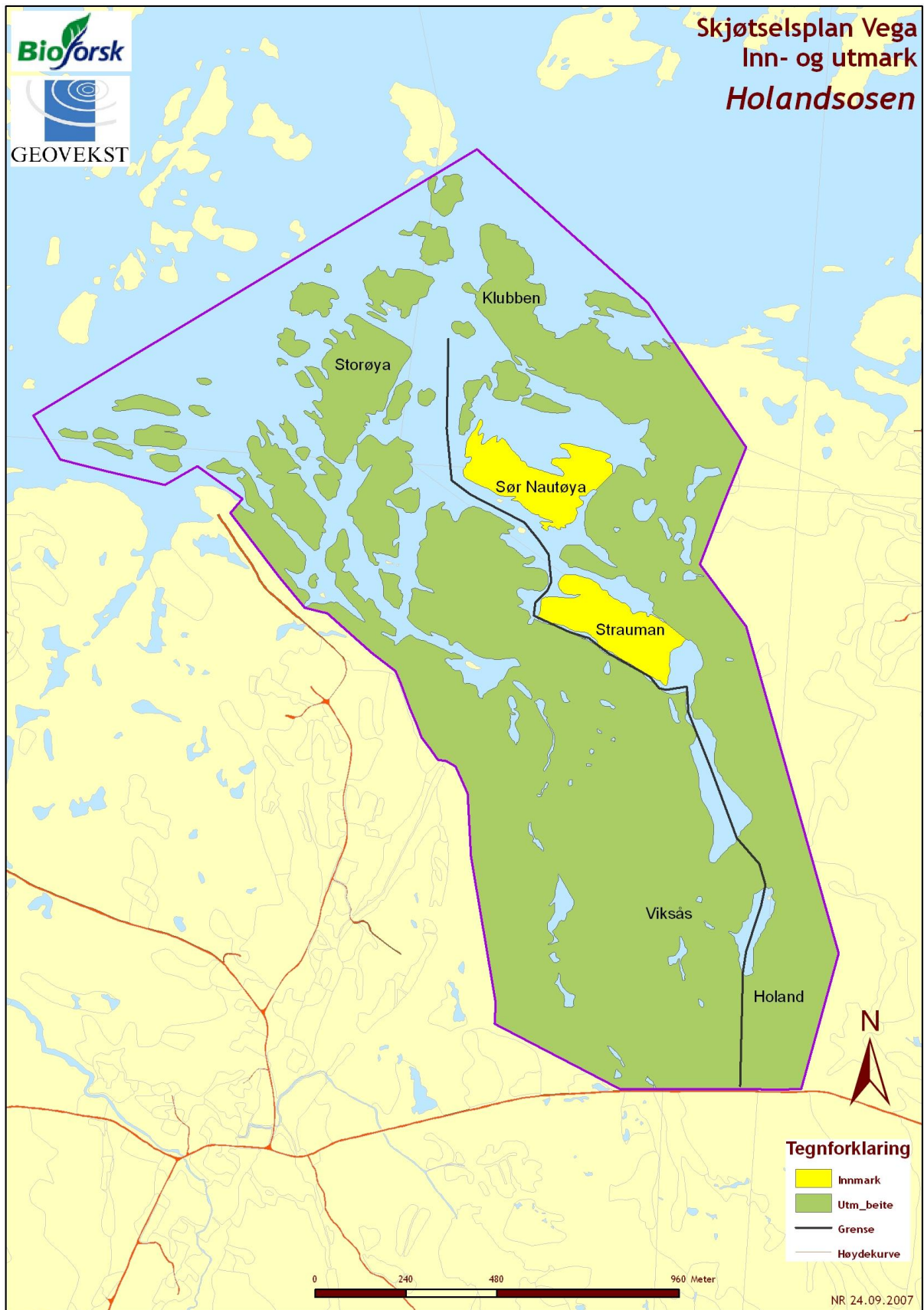
Figur 2. Oversiktskart over tidligere inn- utmarksområder i Holandsosena NR. Hovedsakelig ble området benyttet til felles utmarksbeite. På kartet vises også grensen mellom Viksås- og Holandsida som delvis gikk gjennom osene (Øverosen, nederst mot riksveien og Nerosen, nord for denne).
