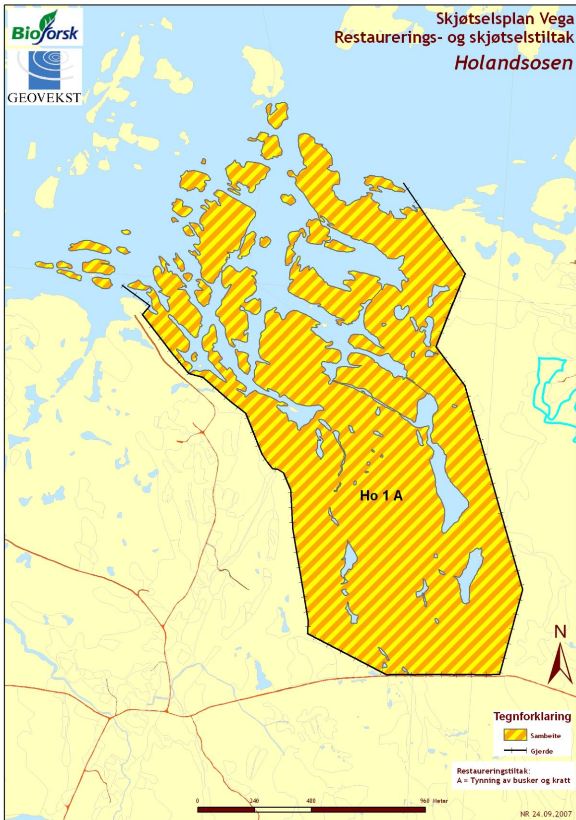
Figur 4: Kart over restaurerings- og skjøtselsforslag i Holandsosen. Gjerdeforslaget følger naturreservatgrensa. Det legges opp til å finne en praktisk og fornuftig løsning på hvor gjerdet bør settes opp, gjerne med utvidelse av området.
