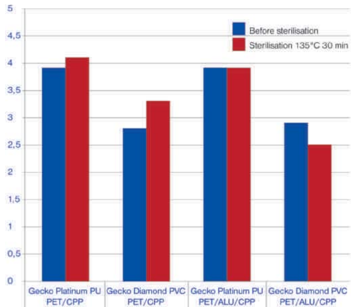
Verbundwerte von Gecko Platinum im Vergleich zu PVC-Farben.
