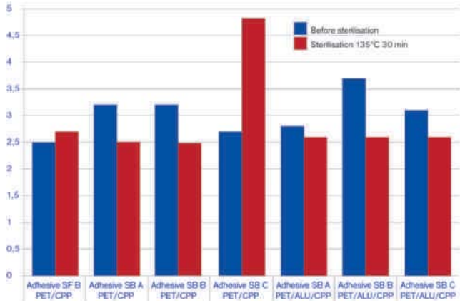
Verbundwerte von Gecko Platinum Flexo mit PET/CPP und PET/Alu/CPP.
