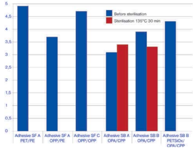
Verbundwerte Gecko Platinum Flexo mit Polyolefinfolien, OPA und PETSIOx.
