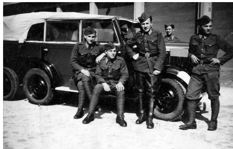
Veliteľský automobil Praga AV od Pluku útočnej vozby. Na blatníku má zástavku predpísanú pre veliteľa pluku. (AM-SNP)
