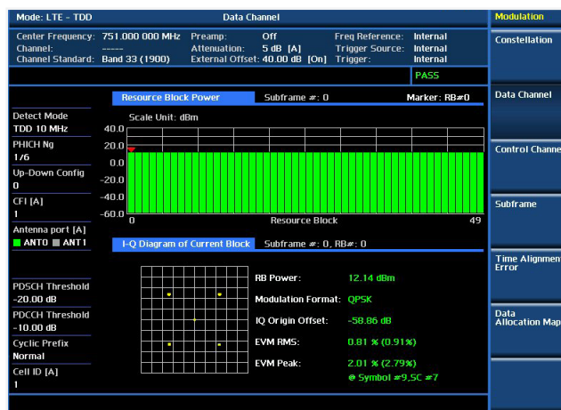
Análisis de modulación: canales de datos
