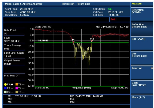
Prueba de cable y antena: reflexión
