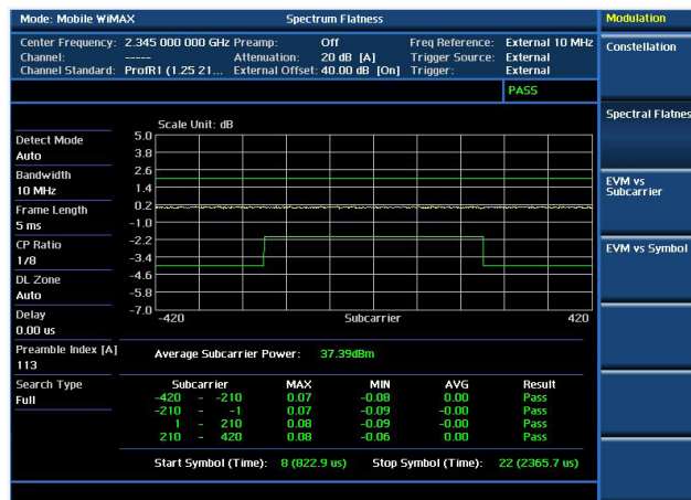
Análisis de modulación: monotonía espectral
