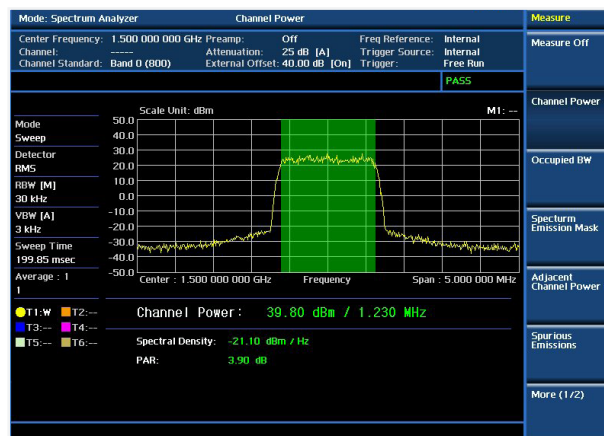
Prueba RF: potencia del canal
