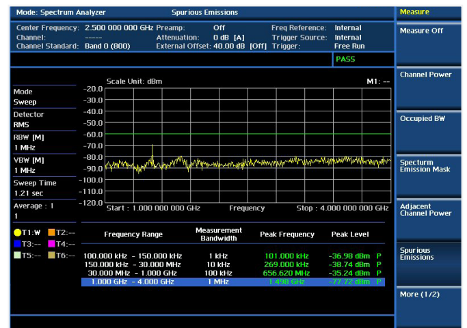
Prueba RF: emisiones espurias
