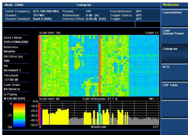
Análisis de modulación: codograma
