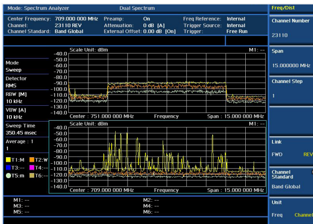
Prueba RF: espectro dual
