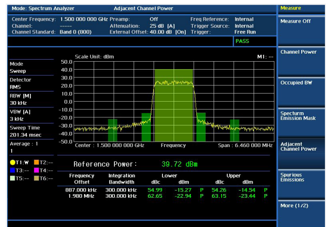
Análisis RF: potencia de canal adyacente
