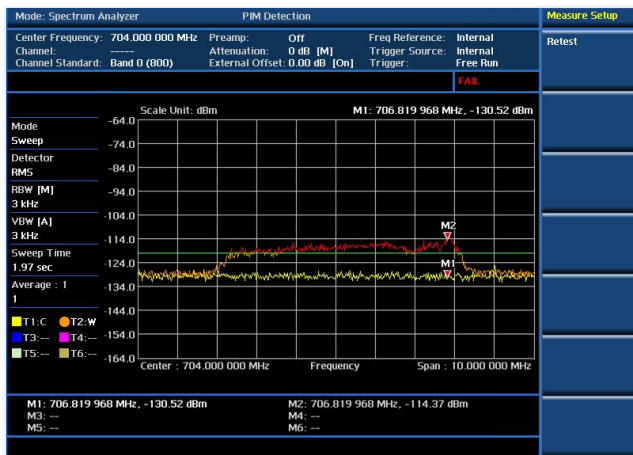
Prueba RF: detección de PIM
