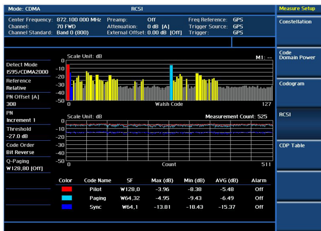
Análisis de modulación: RCSI
