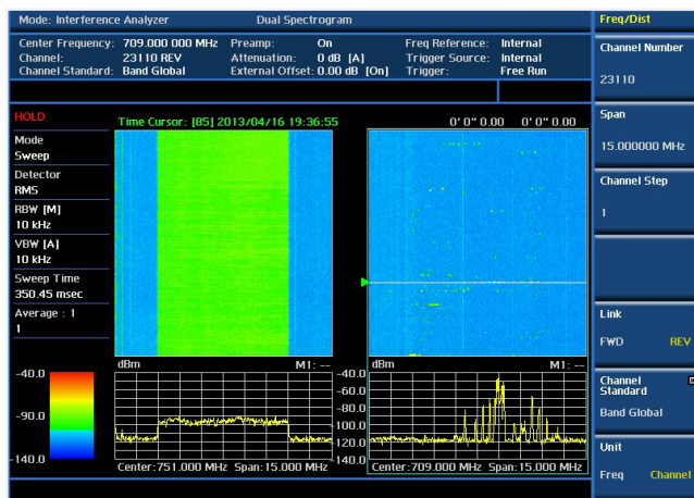
Prueba de análisis de interferencia: espectrograma dual
