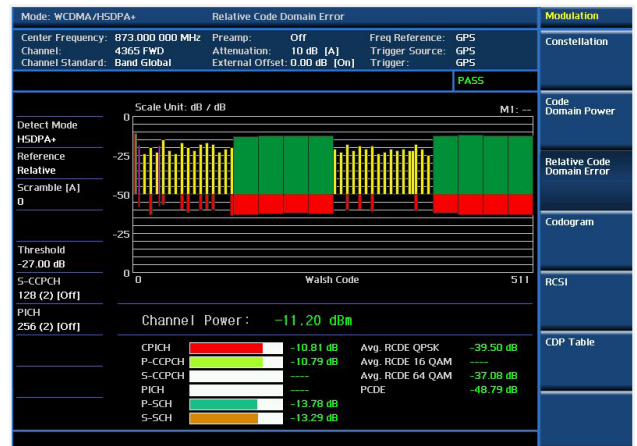
Análisis de modulación: error de dominio de código relativo
