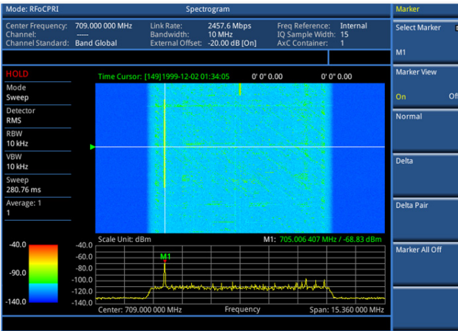
RFOCPRI: espectrograma
