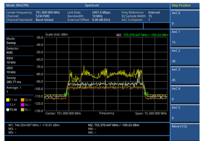
RfOCPRI: espectro
