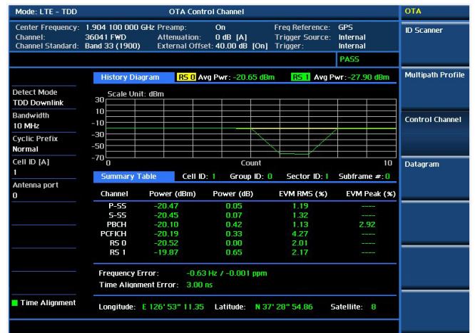
Análisis OTA: canales de control
