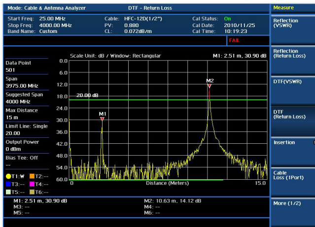
Prueba de cable y antena: distancia a la falla
