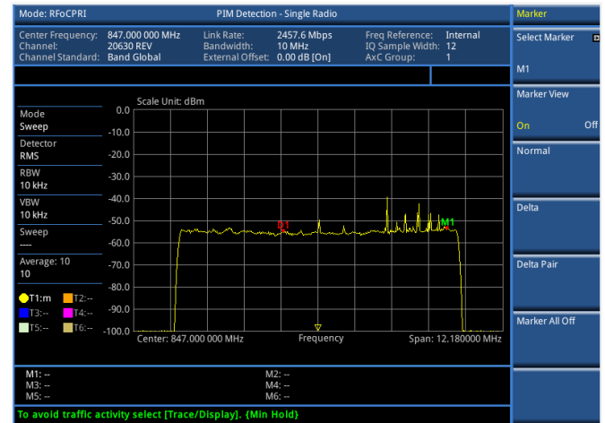
RFOCPRI: detección de PIM
