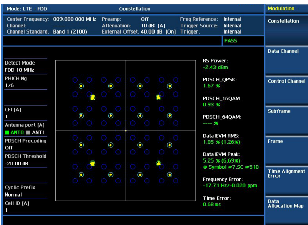
Análisis de modulación: constelación de datos
