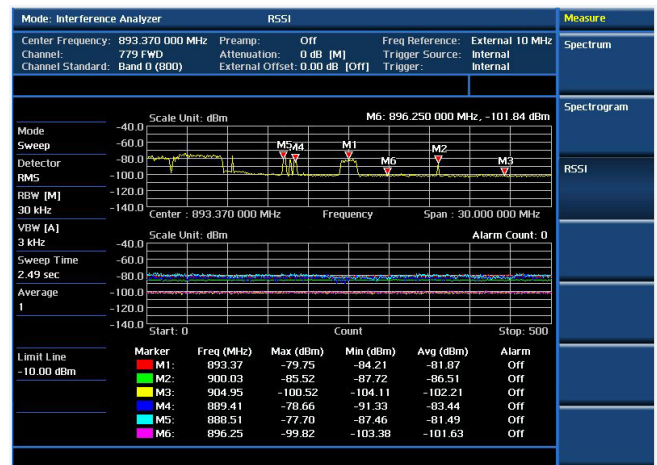
Prueba de análisis de interferencia: RSSI
