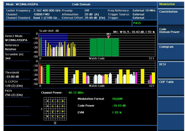
Análisis de modulación: potencia de dominio de código
