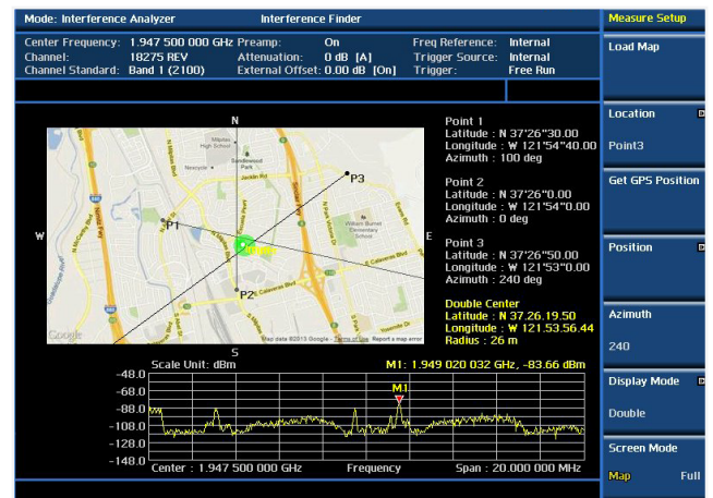
Prueba de análisis de interferencia: buscador de interferencia
