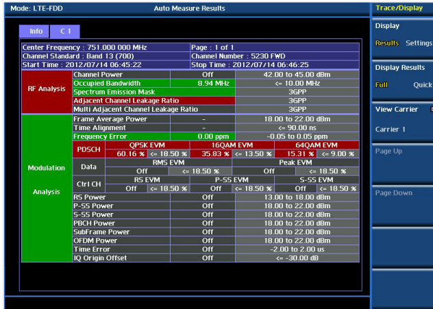
Análisis de modulación y RF: medición automática
