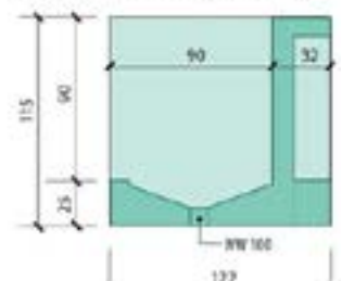
Querschnitt (Ausführung frostsicher)
