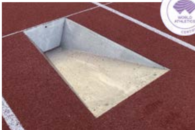
Pole vault puncture box „Default“
