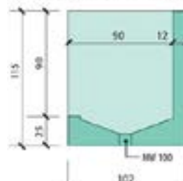
Querschnitt (Normalausführung)
