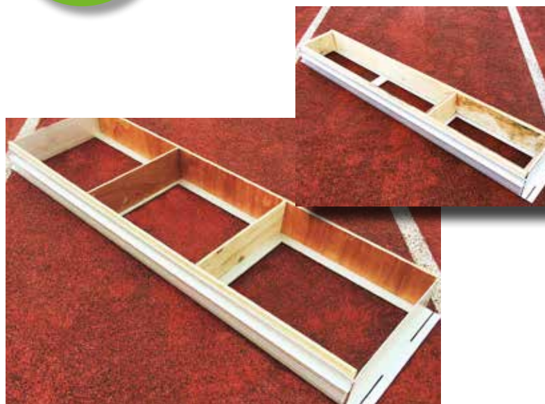
Foundation tray „Standard“ 122/34/10 cm
