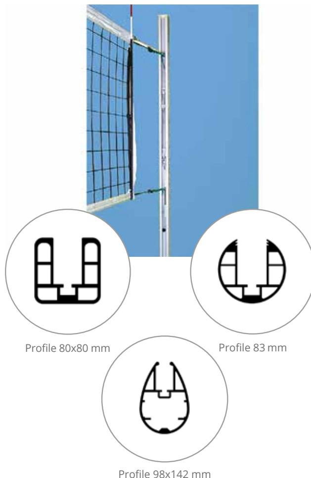
Profil 98x142
