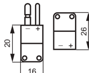
Miniature plugs
