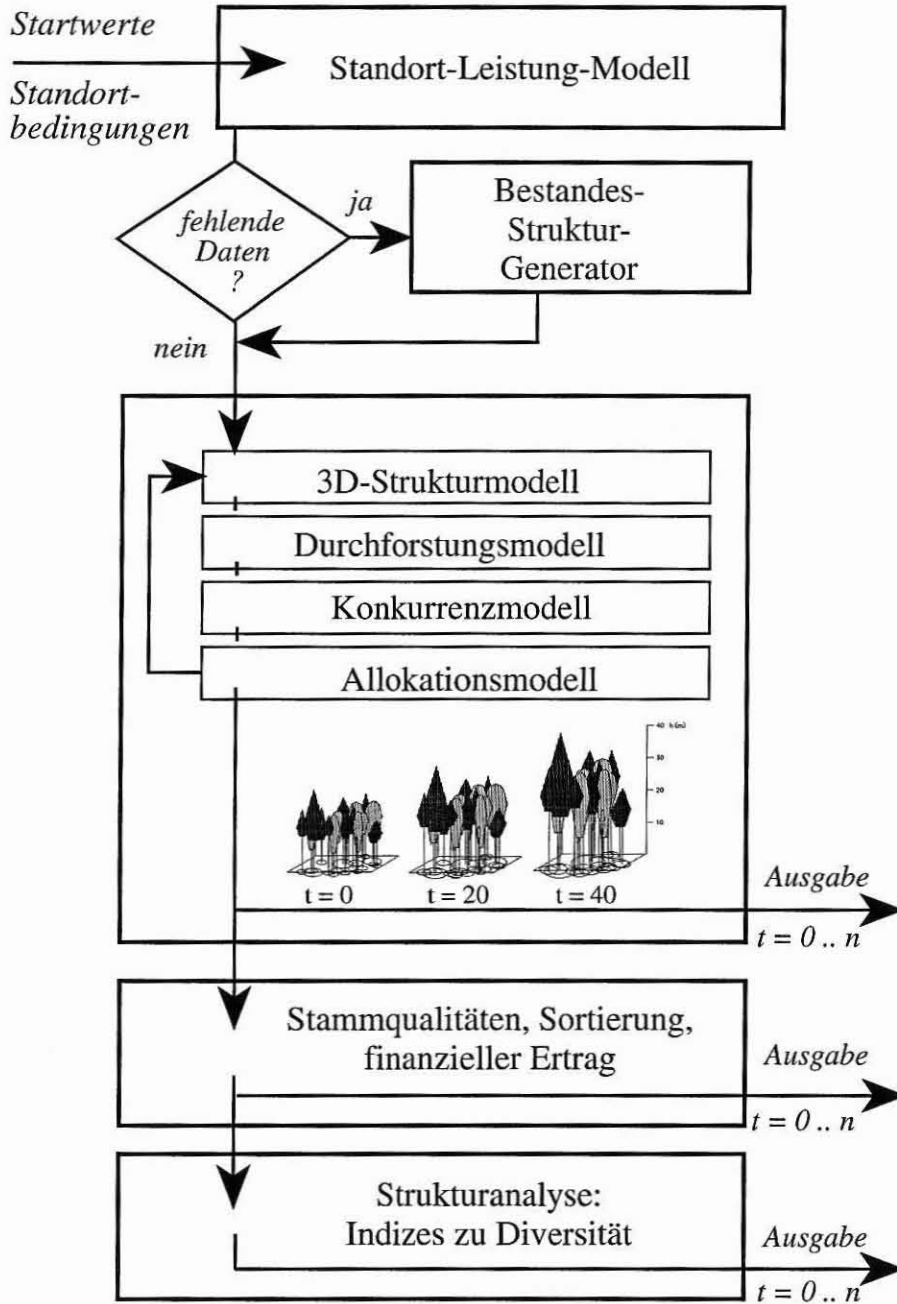
Abb. 5: Algorithmischer Ablauf des Bestandeswachstummodells SILVA 2 mit Programmroutine zur Strukturanalyse.
