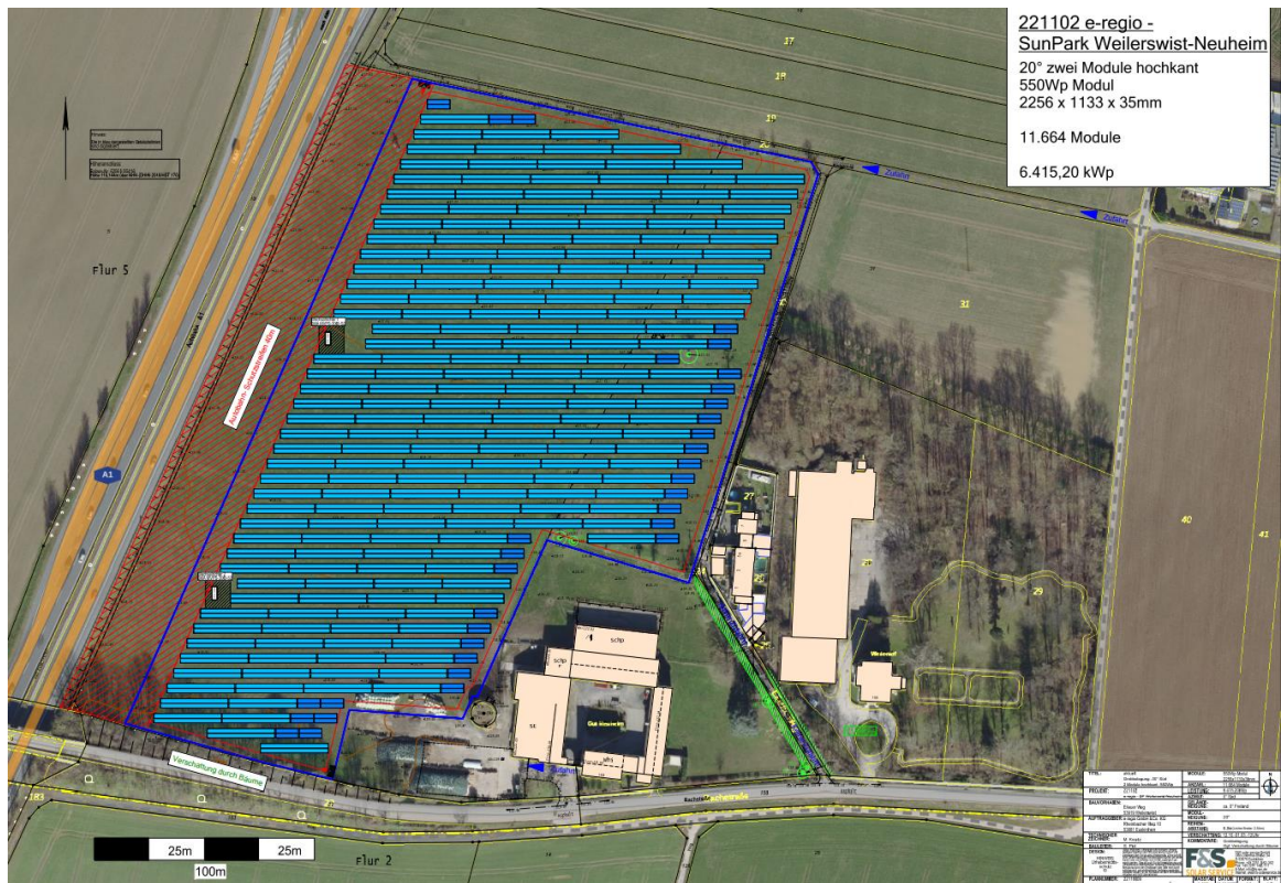
Abbildung 2: Grobbelegung
