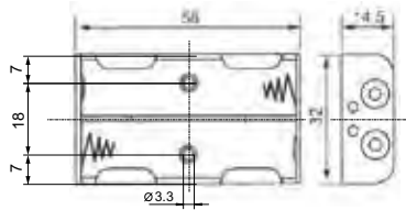
Goobay 2x AA (Mignon) Batteriehalter Lötflanke (U)
