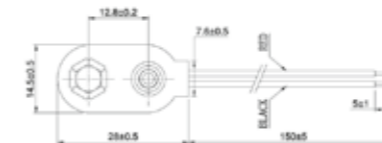
Goobay 1x 9V Block Batteriehalter Lose Kabelenden
