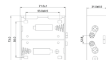
Goobay 2x D (Mono) Batteriehalter Druckknopf
