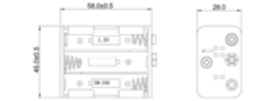
Goobay 6x AA (Mignon) Batteriehalter Druckknopf
