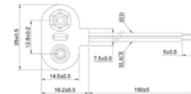
Goobay 1x 9V Block Batteriehalter Lose Kabelenden
