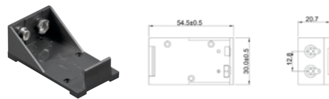
Goobay 1x 9V Block Batteriehalter Lötflanke (U)
