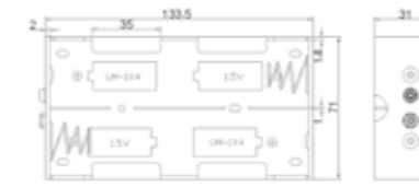
Goobay 4x D (Mono) Batteriehalter Druckknopf
