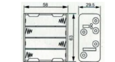
Goobay 8x AA (Mignon) Batteriehalter Lose Kabelenden
