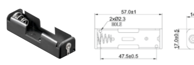
Goobay 1x AA (Mignon) Batteriehalter Lötfläche (U)
