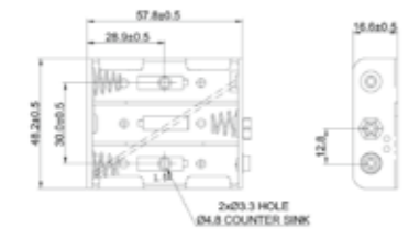
Goobay 3x AA (Mignon) Batteriehalter Druckknopf
