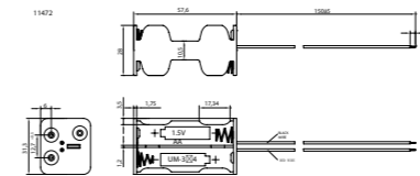
Goobay 4x AA (Mignon) Batteriehalter Lose Kabelenden
