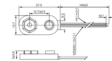
Goobay 1x 9V Block Batteriehalter Lose Kabelenden, wasserabweisend
