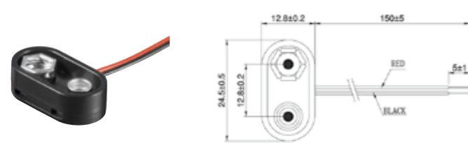
Goobay 1x 9V Block Batteriehalter Lose Kabelenden, wasserabweisend
