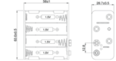
Goobay 8x AA (Mignon) Batteriehalter Druckknopf
