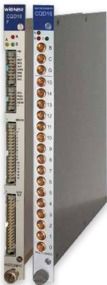
CQ16 (left) and CQ16A Module
