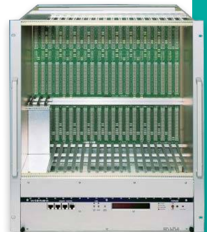
9U VME 6023 Crate
