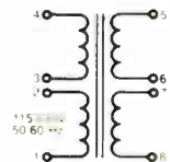
8 PIN TYPE D5T
