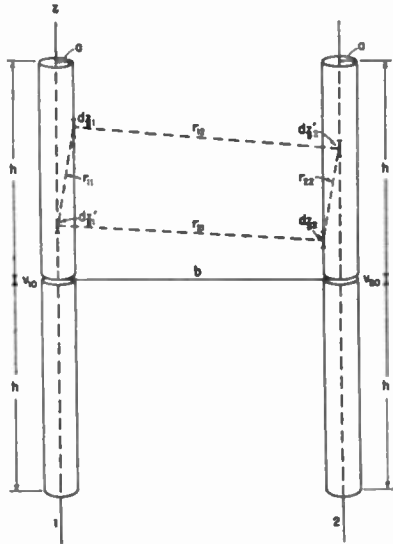
Fig. 1—Two coupled antennas.
