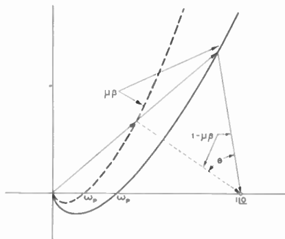
Fig. 5—Phase shift of 1 - \mu\beta .
