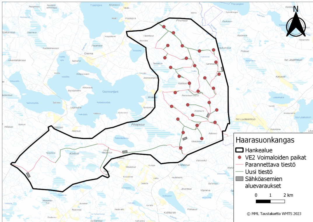
Kuva 3. Haarassuonkankaan tulivoimapuiston alustava voimalasijoittelu vaihtoehdossa VE2.
