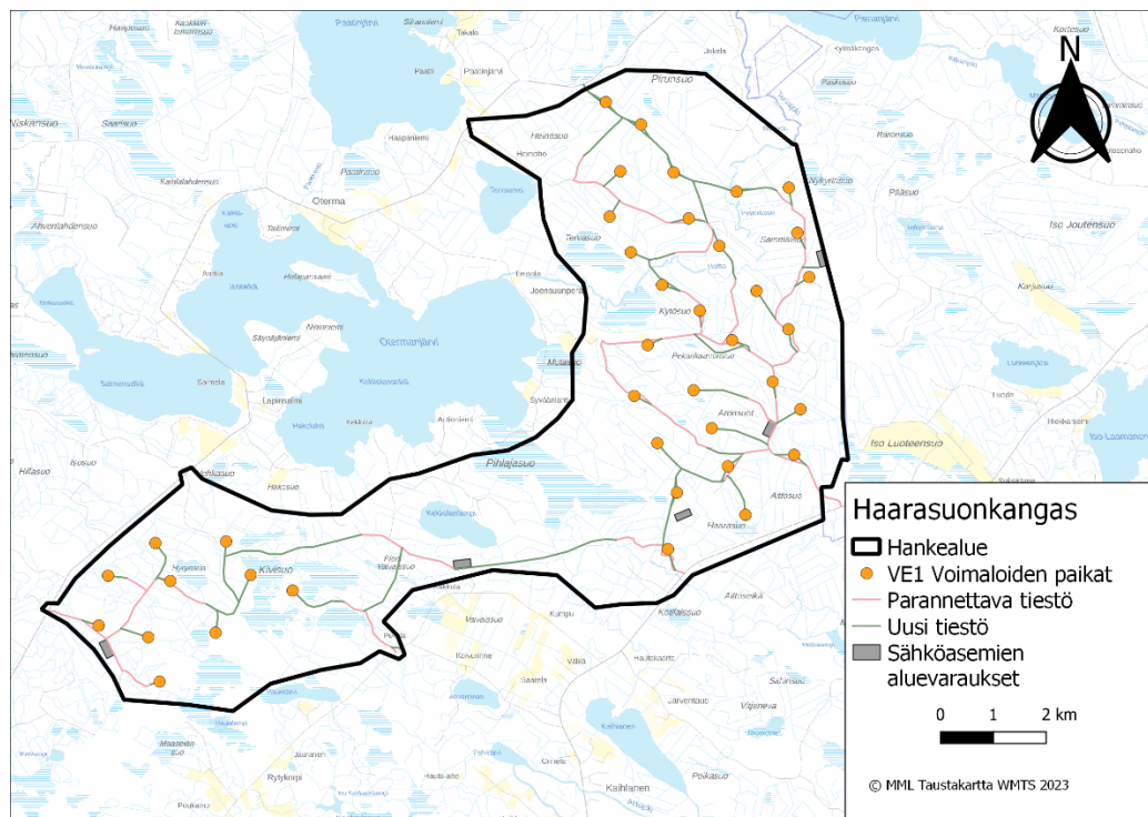
Kuva 2. Haarasuonkankaan tuulivoimapaiston alustava voimalasijoittelu vaihtoehdossa VE1.
