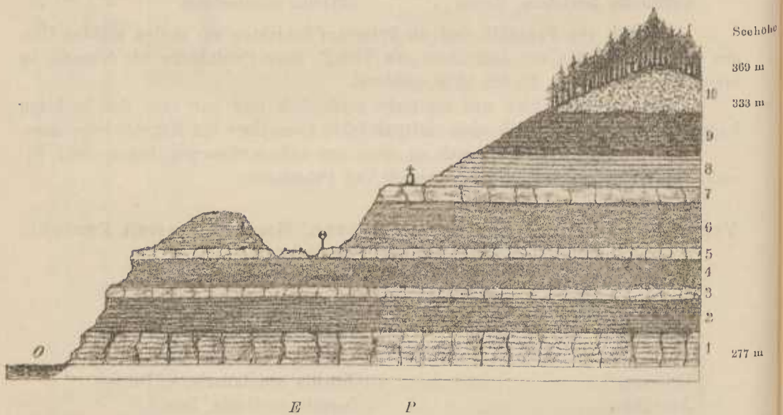
Fig. 27. Profil der Berglehne „Sutiny“ bei Chotzen.
