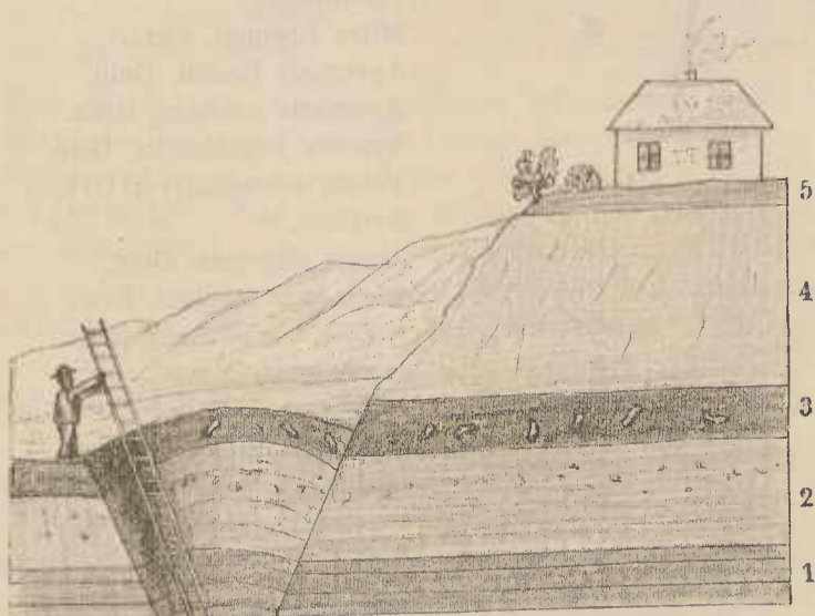
Fig. 25. Profil in der Ziegelei bei Mikulovie bei einer behufs Wassergewinnung angelegten Grube. 1. Tiefere Lage der Teplitzer Schichten mit Lima elongata . 2. Höhere Lage der Teplitzer Schichten mit Rhynchonella octoplicata . 3. Tiefste Lage der Priesener Schichten mit stammförmigen Concretionen. 4. Gelber Ziegellehm. 5. Ackerkrume.
