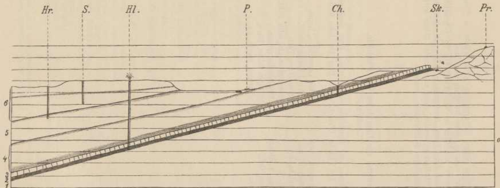
Fig. 28. Schematisches Profil in der Richtung von Chrudim gegen Königgrätz, das Verhältniss der wasserführenden Schichten der Kreideformation darstellend.
