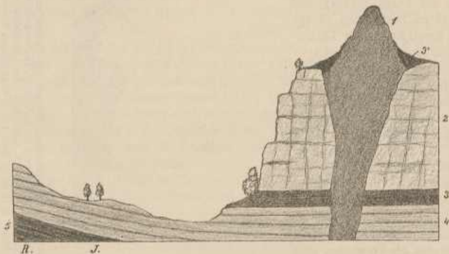
Fig. 21. Ideales Profil der Trosky gegen Rovensko (R.) hin.
