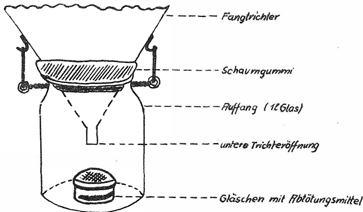
Fig. 14. Insekten-Auffang mit Gläschen für Abtötungsmittel für die nach MESSCH veränderte Form der Minnesota-Lichtfalle
