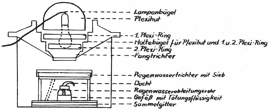
Fig. 1. Die verbesserte Robinson-Lichtfalle nach RUSSELL (1960)
