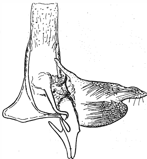
Fig. 180. Infurcitinea marcunella (Rbl.). ♂ Genitalapparat, aufgeklappt. Eine Valve entfernt.
