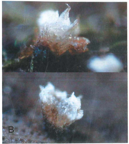
Abb. 1: Coronellaria pulicaris (A: Oploo, H.B. 6855; B: Potsdam, H.B. 6730a); A - Blick auf Ectalexipulum (KOH), B - Habitus eines Apotheciums (rehydriert). Fotos: H.-O. BARAL.
