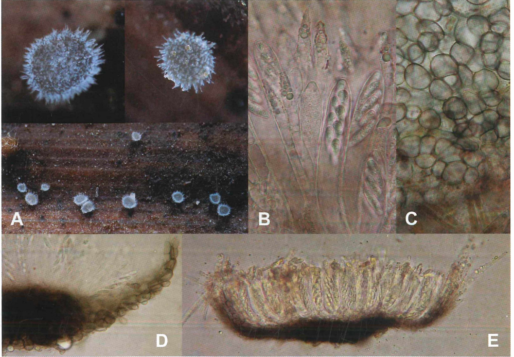
Abb. 4: Coronellaria caricinella (Rehna, H.B. 8471a); A - Habitus der Apothecien (frisch), B - Asci und Paraphysen (vital), C - Blick auf Ectalexciplum (vital), D, E - Medianschnitte (KOH). Fotos H.-O. BARAL.
