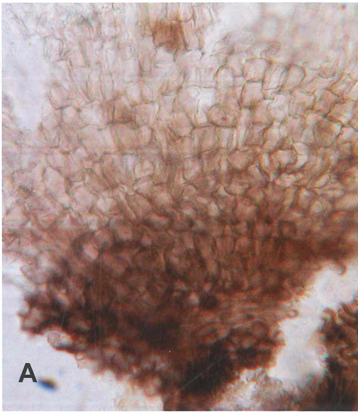
Abb. 1: Coronellaria pulicaris (A: Oploo, H.B. 6855; B: Potsdam, H.B. 6730a); A - Blick auf Ectalexipulum (KOH), B - Habitus eines Apotheciums (rehydriert). Fotos: H.-O. BARAL.
