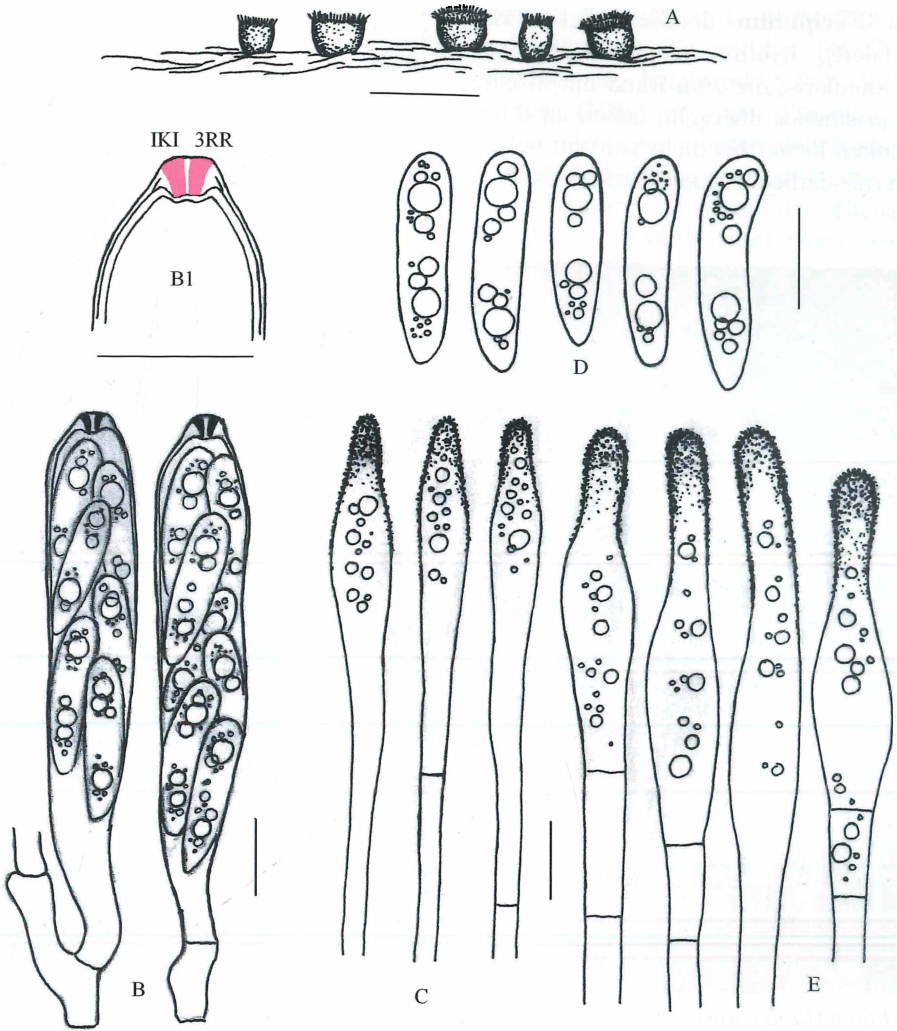
Abb. 3: Coronellaria spec. (Gr. Pälitzsee, H.B. 8405); A – Habitus, Apothecien vergrößert, B – Ascus: B1 – Ascusapex mit Apikalring (tot), C – Paraphysen (vital), D – Ascosporen mit Lipidtropfen (vital), E – Haare. Maßstäbe: A= 1 mm; B-D= 10 \mu m – Zeichnung: T. RICHTER.
