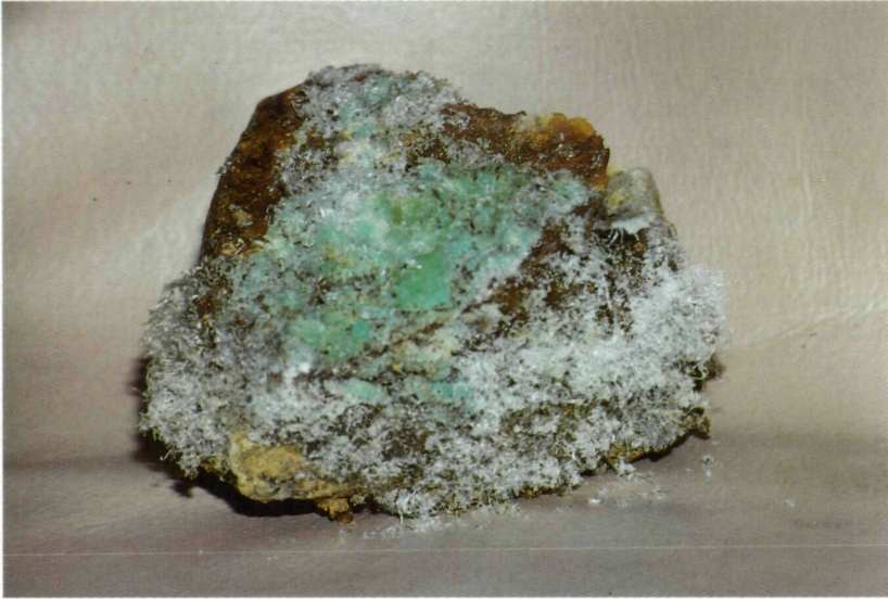
Abb. 3: Grünblaue Ausblühungen von Siderotil auf Pyrit; Maßstab 1:1; Fundort: Lading. Foto und Sammlung: M. PUTTNER
