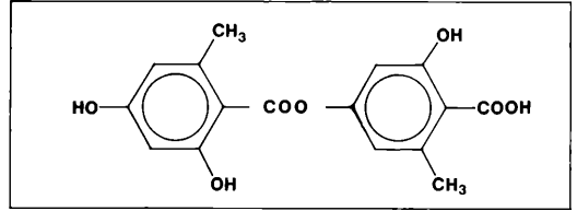
Abbildung 1. Lecanorsäure.
