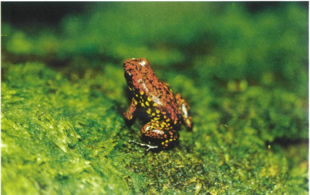
Fig. 7: Dendrobates occultator from Quebrada Guanguí, Colombia (population 6). Abb. 7: Dendrobates occultator vom Quebrada Guanguí, Kolumbien (Population 6).
