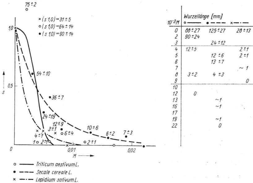
Abb. 5. s in Abhängigkeit von M bei OAS im Schadstofftest. Näherungsgleichungen der dargestellten Kurven
