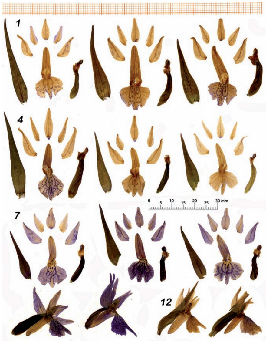
Abb. 27: D. urvilleana , Blütenanalysen, West-Georgien. Fig. 1-6: Kartli, Rikotipaß, 890 m, 28.5.2004, Lo 04.118; fig. 7-11: Ratscha, Nikorzmina, 1160 m, 31.5.2004, Lo 04130d. Leg. MA, RL, MM.
